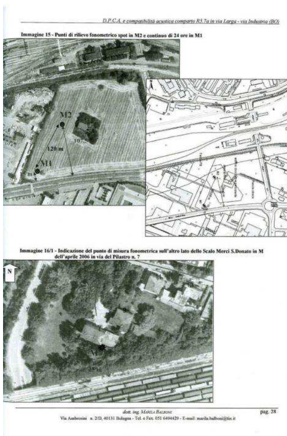
Figura 4 - Dati acustici reperiti dalla DPCA del comparto R5.7a
